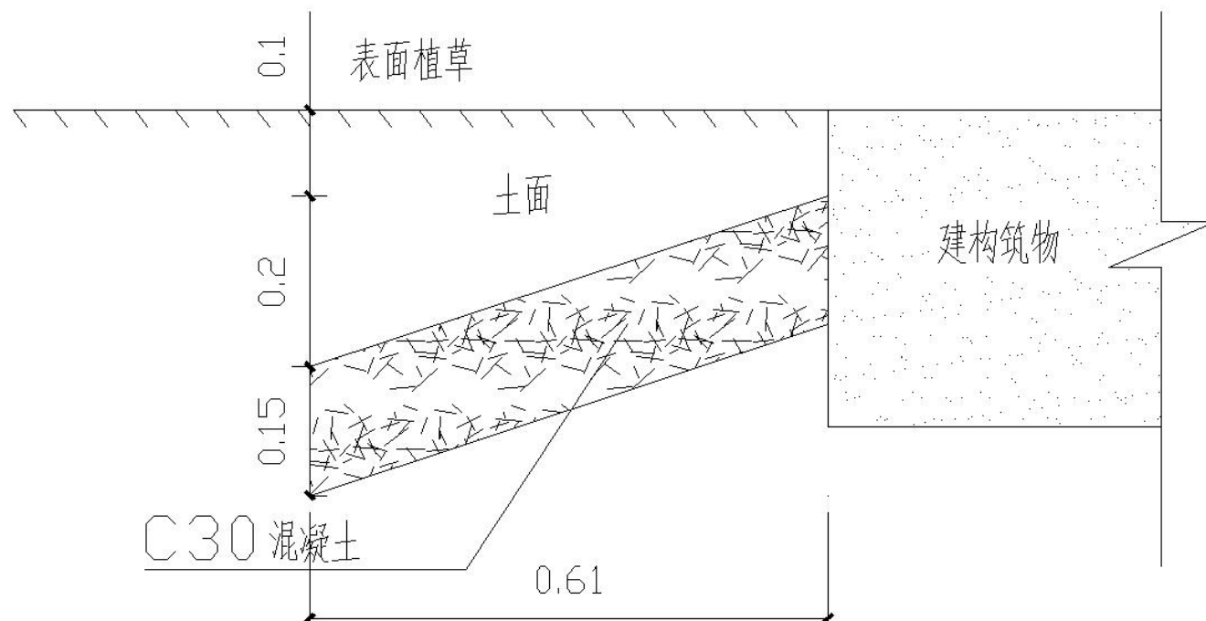
直立面消除剖面示意图
