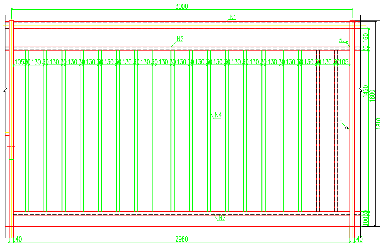
栏杆立面图
